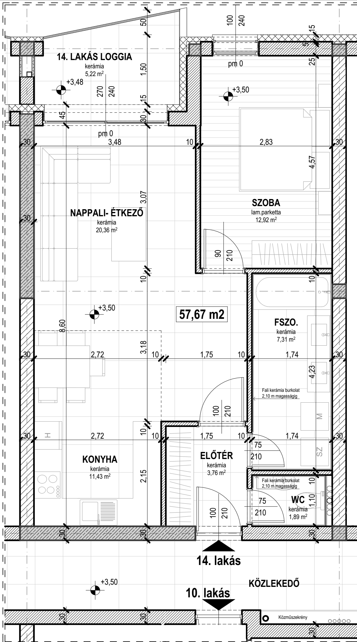
HAJDÚSZOBOSZLÓ, SZURMAI UTCA 4-6. SZ. - EMELET - 14. LAKÁS - 57,67 m 2
